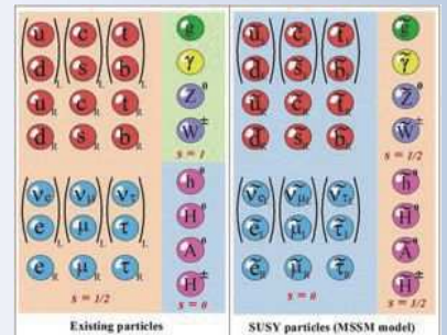
素粒子と超対称パートナー
