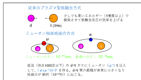
▲ミューオン触媒核融合方式
