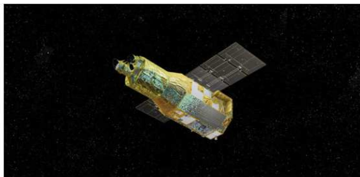
2023 年 9 月に打ち上げられた日本の X 線天文衛星 XRISM
