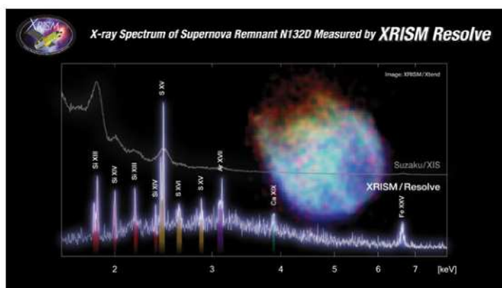
XRISM が観測した超新星残骸 N132D の X 線分光スペクトル
