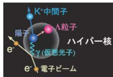
電子ビームを使ってハイパー核を生成し、K中間子と電子(e)を同時測定することで100億分の2秒しか存在しないハイパー核の質量を知ることができます。
