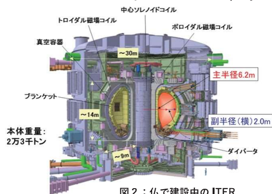
図2：仏で建設中のITER （国際熱核融合実験炉, International Thermonuclear Experimental Reactor） の鳥瞰図
